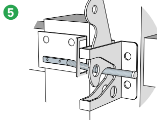
Loquet installé à l'intérieur de l'enceinte
